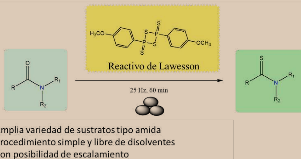
Esquema 1. Síntesis mecanoquímica del segmento de tioamida con el reactivo de Lawesson.
